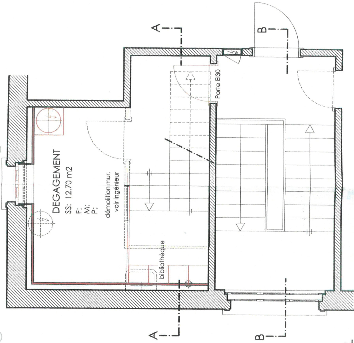
2ème ETAGE PARTIEL
